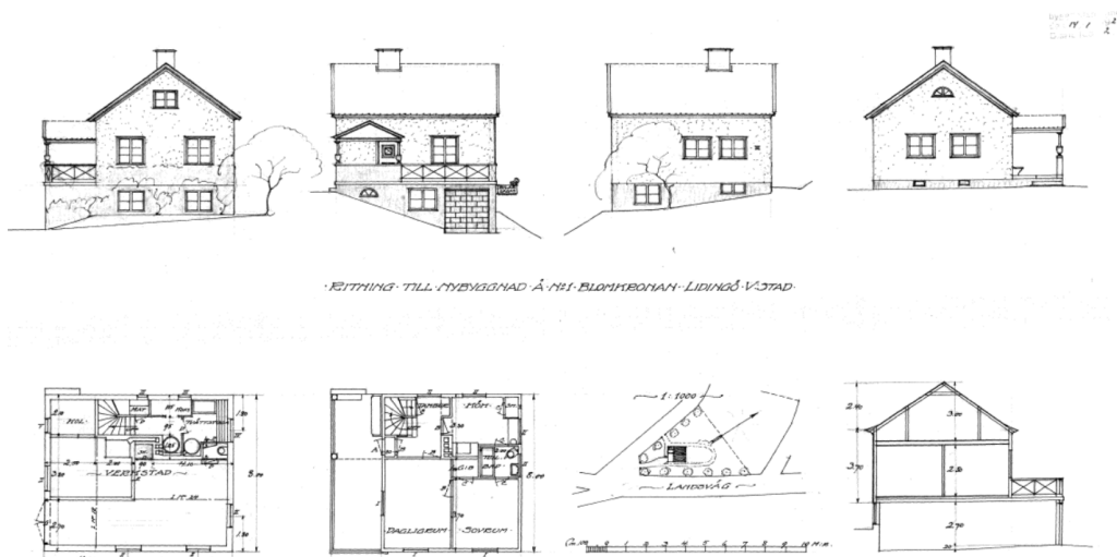
Ritningar från ursprungsbygglov 1926.
