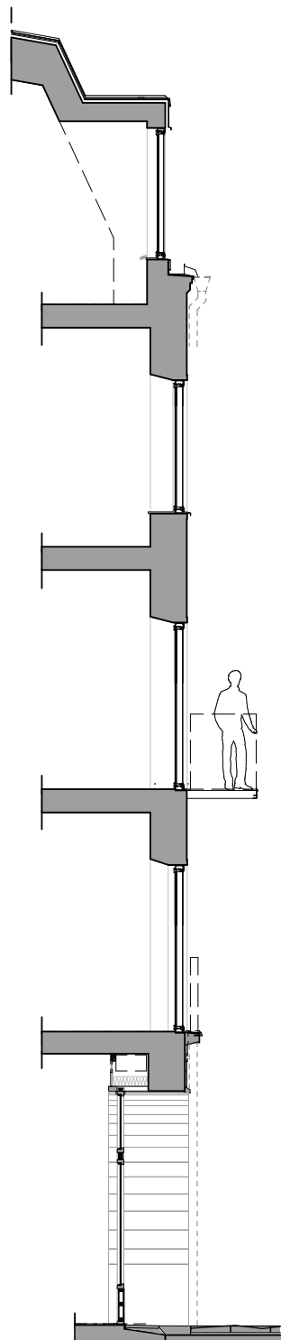
Sektion. Bild: Brunnberg och Forshed.
