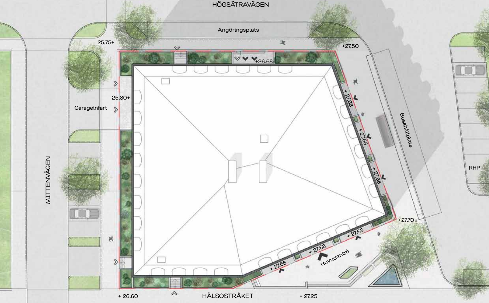
Illustrationsplan för Hälsans hus. Bild: Urbio.
