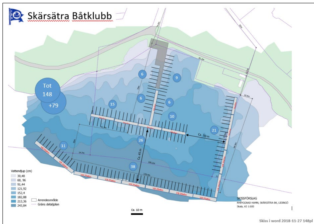
Skissförslag som visar hur nya båtplatser kan kombineras med vågbrytare.
