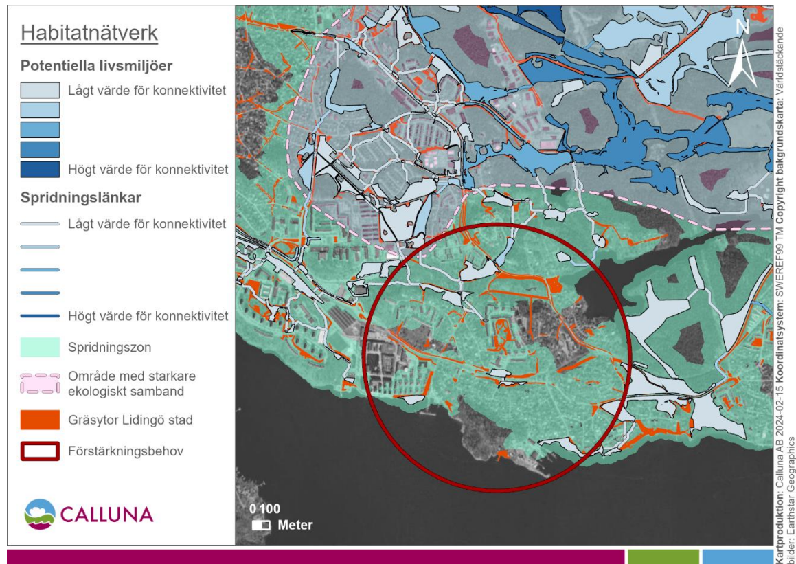
Figur 12. Kartan visar habitatnätverk för pollinatörer i den södra delen av Lidingö. Områden där ett svagare samband kan förstärkas är markerade med en röd ring.
